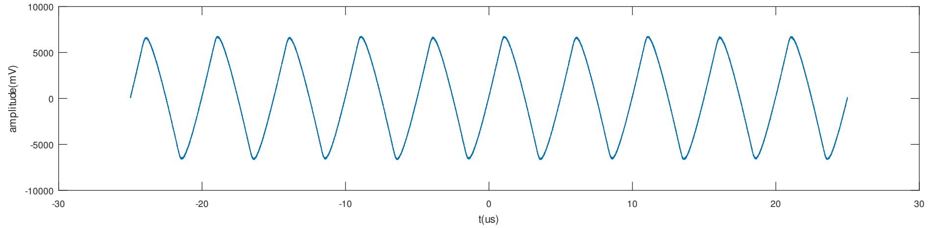
Sinal - Saída f=200kHz do gerador de sinais com ganho maximo
