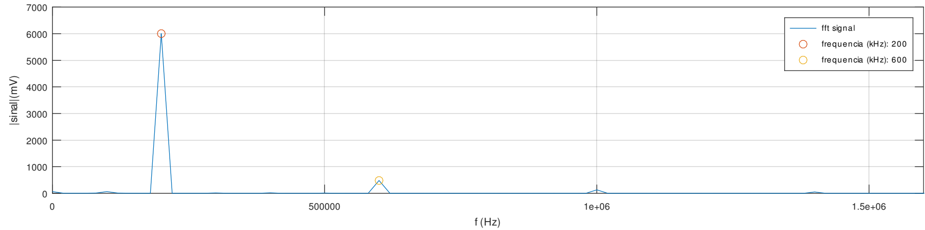
Espectro de amplitudes unilateral X(t) - Saída f=200kHz do gerador de sinais com ganho maximo
